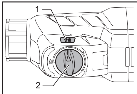
► 1. Rotation avec martelage 2. Bouton de changement de mode
