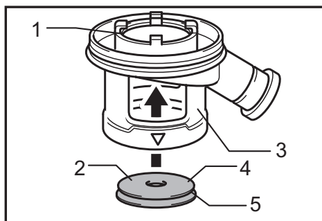
► 1. Bord intérieur 2. Côté plat 3. Dispositif de fixation 4. Bouchon 5. Rainure
