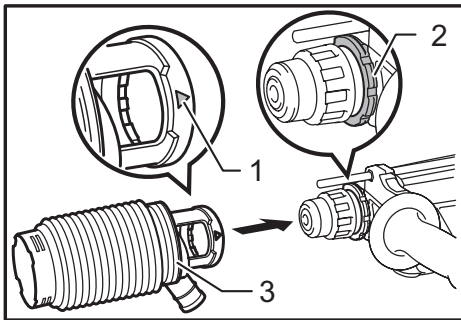
► 1. △ symbol 2. Grooves 3. Dust cup
